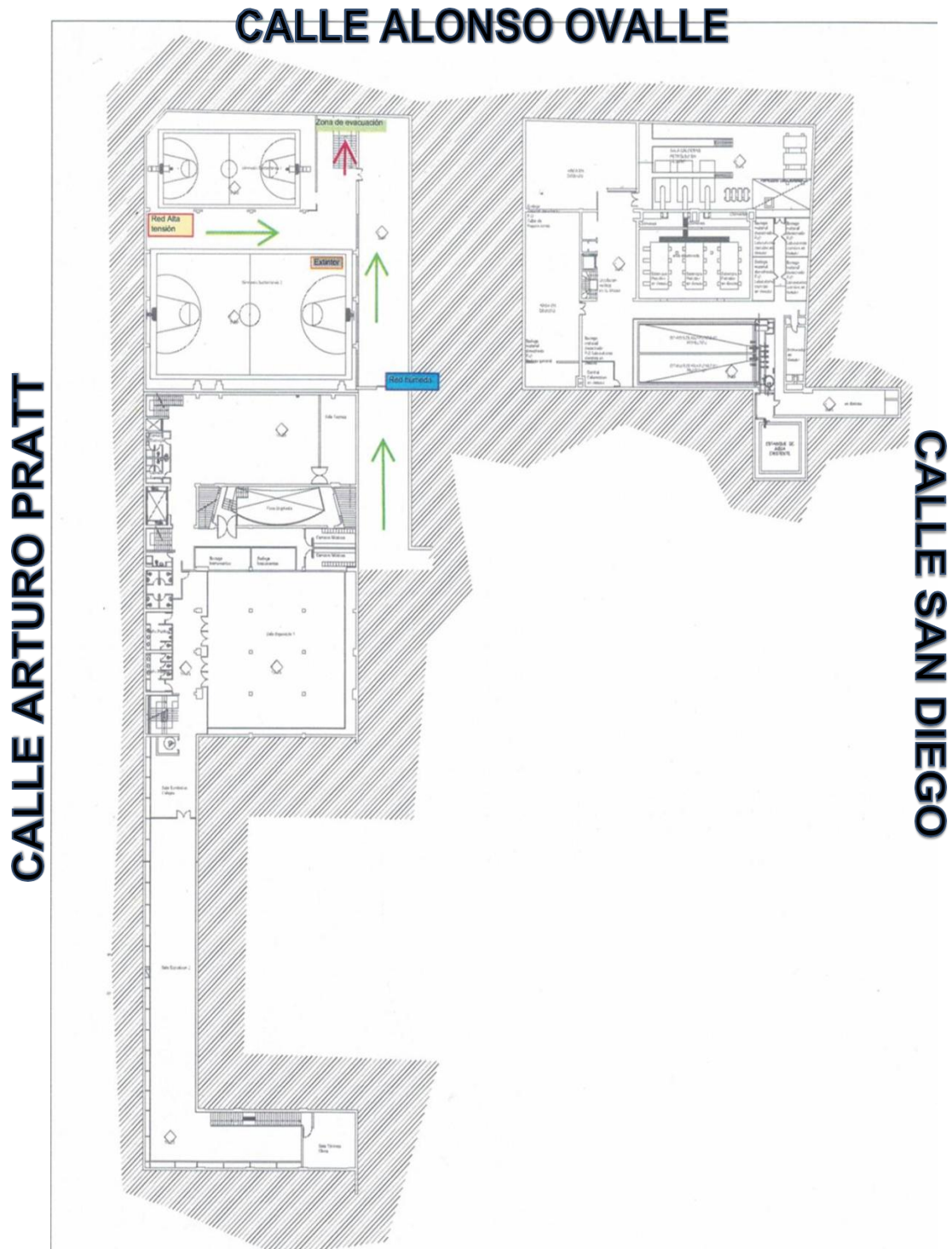
PLANTA SUBTERRANEO ESCALA 1:500
