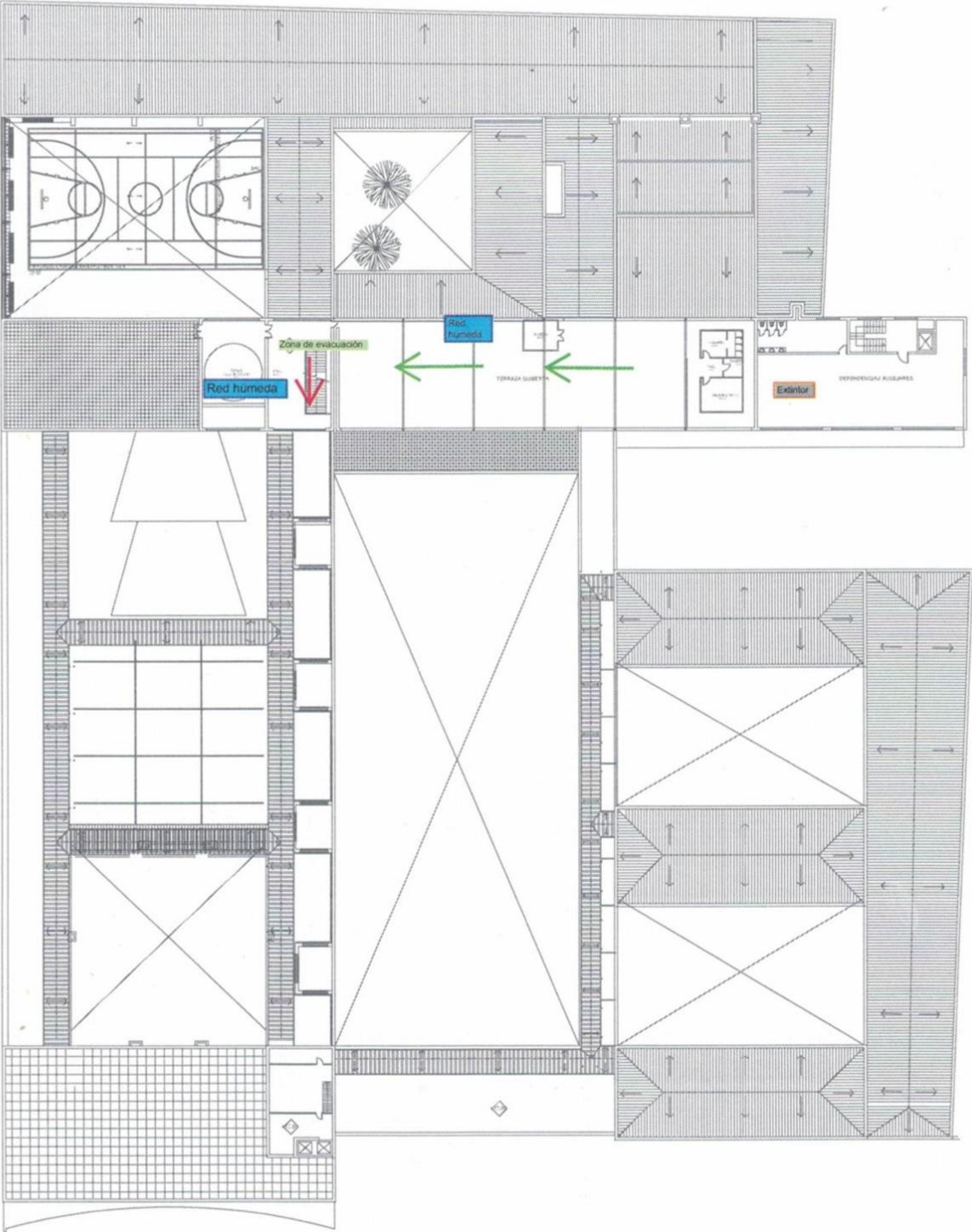
PLANTA TERRAZA ESCALA 1:50
